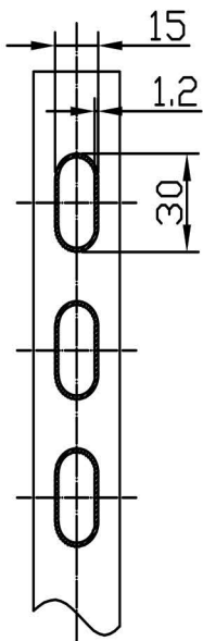
B-B(3:1)
